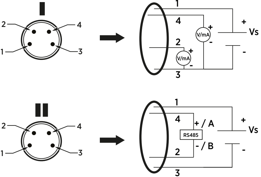
图4 接头引出线
